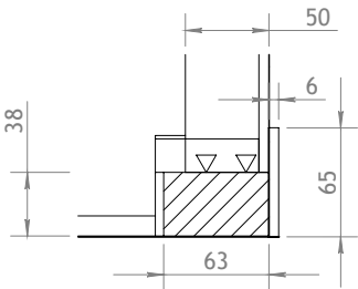
DETAIL Y SCALE 1 : 5
