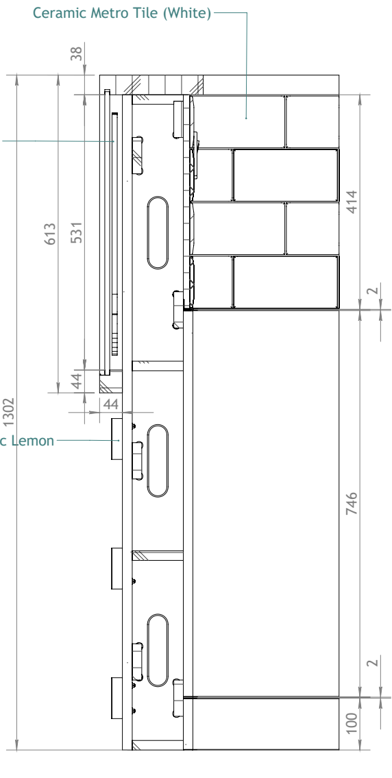
SECTION D-D
